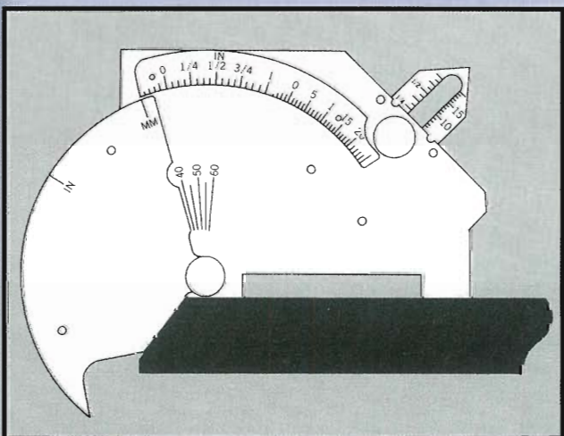
開先角度の測定
