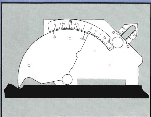
アンダーカット深度測定
