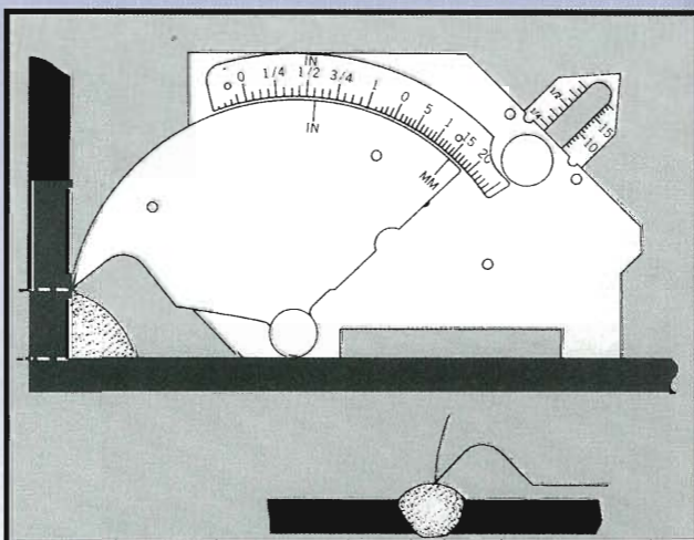
スミ肉部大きさ及ビードの高低の管理
