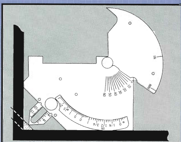
スミ肉部脚長の測定
