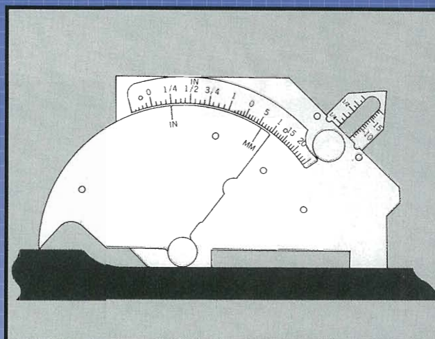
付き合せ材の段差測定
